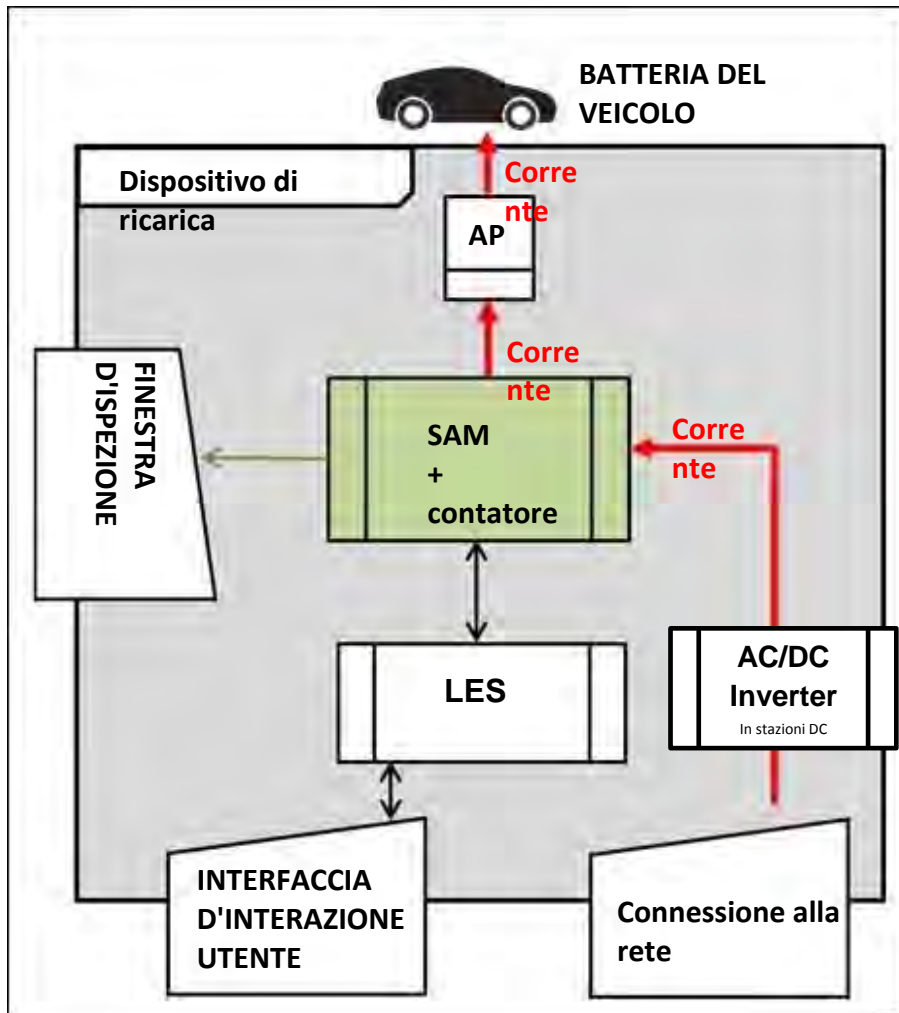
Figura 4: classificazione funzionale del SAM in una stazione di ricarica AC
