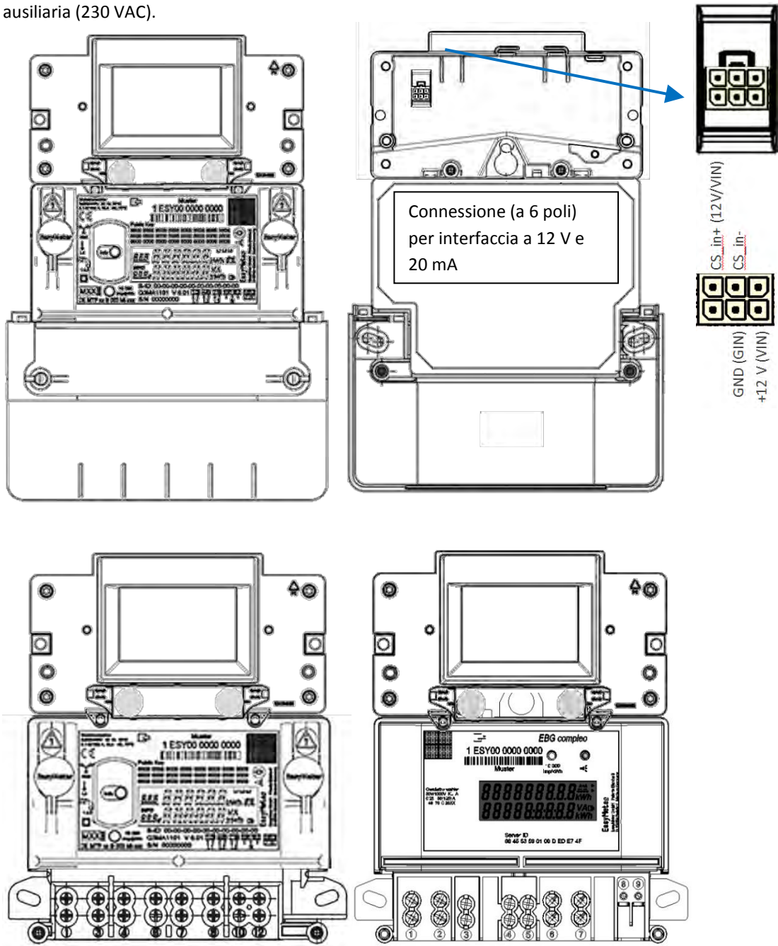
Figura 25: in alto: Fronte e retro con contatore AC, sotto la figura dei terminali; a sinistra AC, a destra DC 1)
