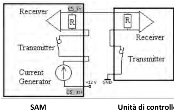
Figura 26: Schema di connessione SAM Interfaccia 20 mA all'unità di controllo
