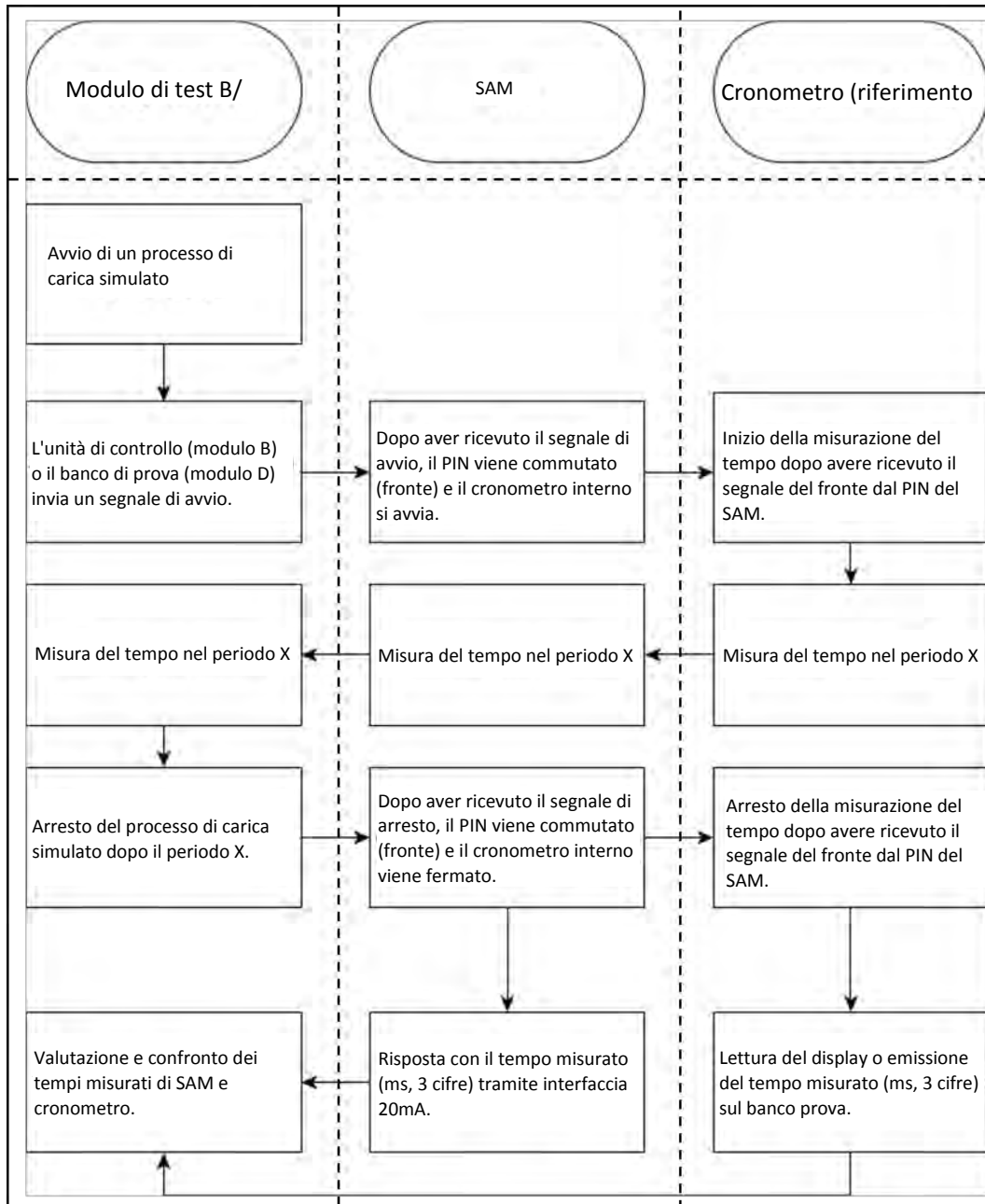
Figura 8: Processo di test relativo alla funzione cronometro nel processo di fabbricazione.
