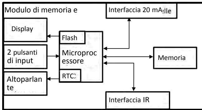
Figura 6: Schema a blocchi funzionale del SAM
