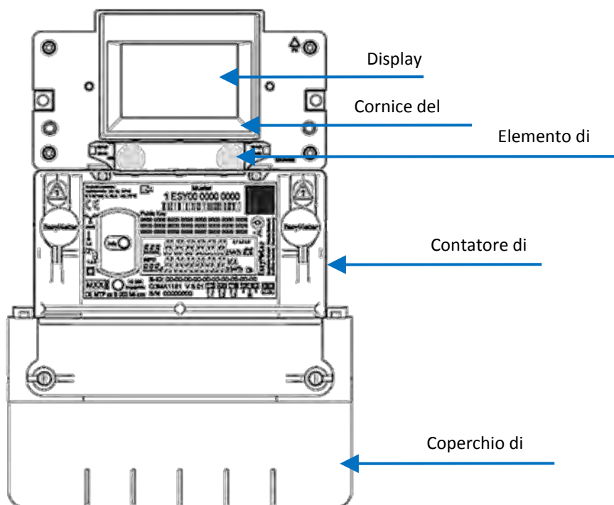
Figura 1: Panoramica del SAM (esempio)
