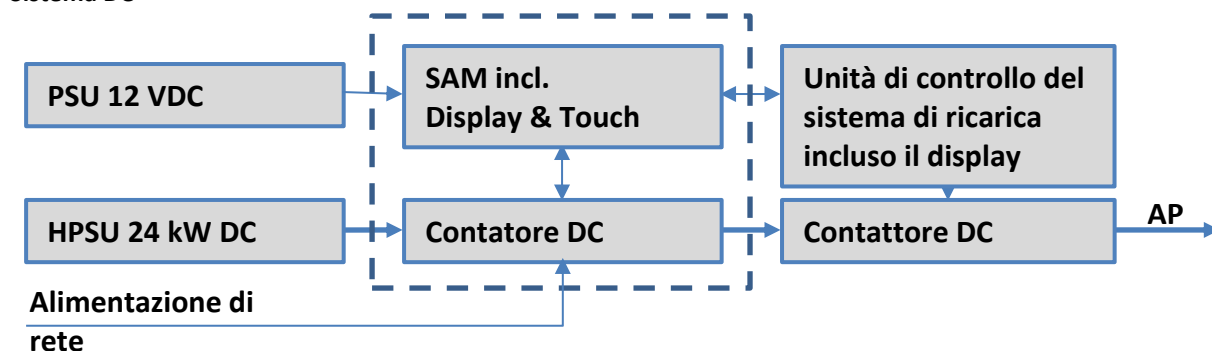
Figura 5: Integrazione del sottosistema in una stazione di ricarica (per variante AC e DC)
